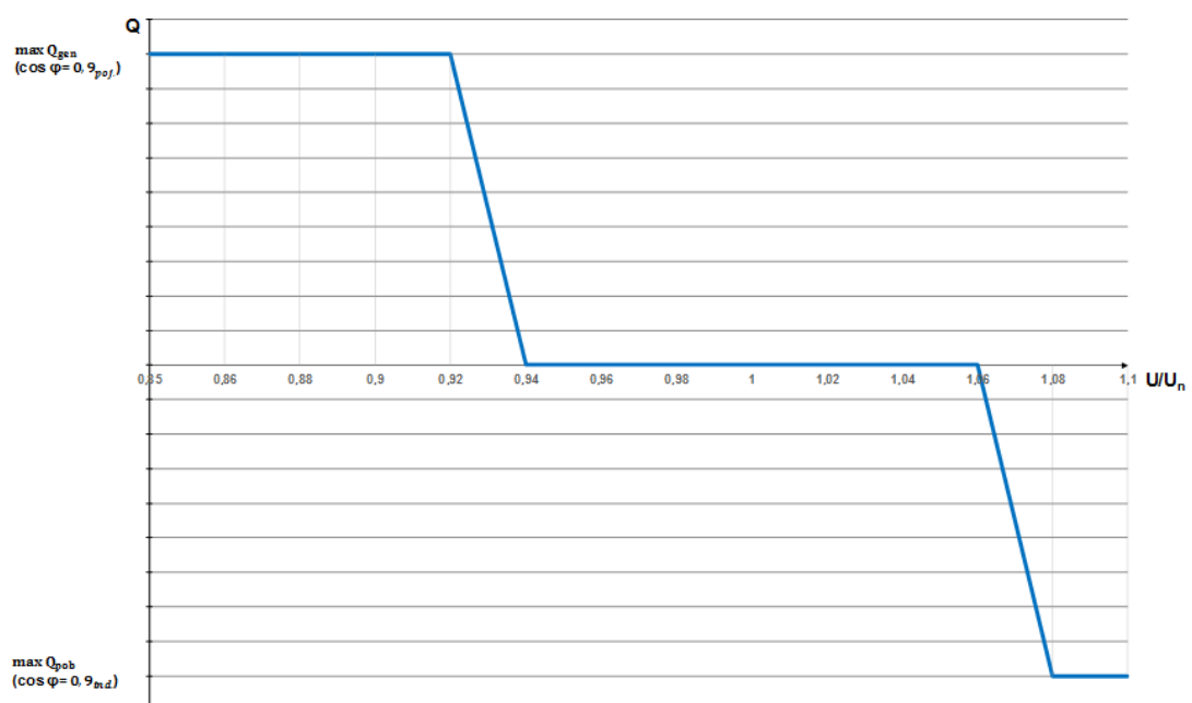
Rys. 3. Charakterystyka sterowania mocą bierną w funkcji napięcia wymagana przez ZEW Niedzica
