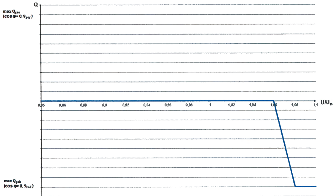
Rys. 4. Charakterystyka sterowania mocą bierną w funkcji napięcia dla mikroinstalacji podłączonych jednofazowo, wymagana przez ZEW Niedzica
