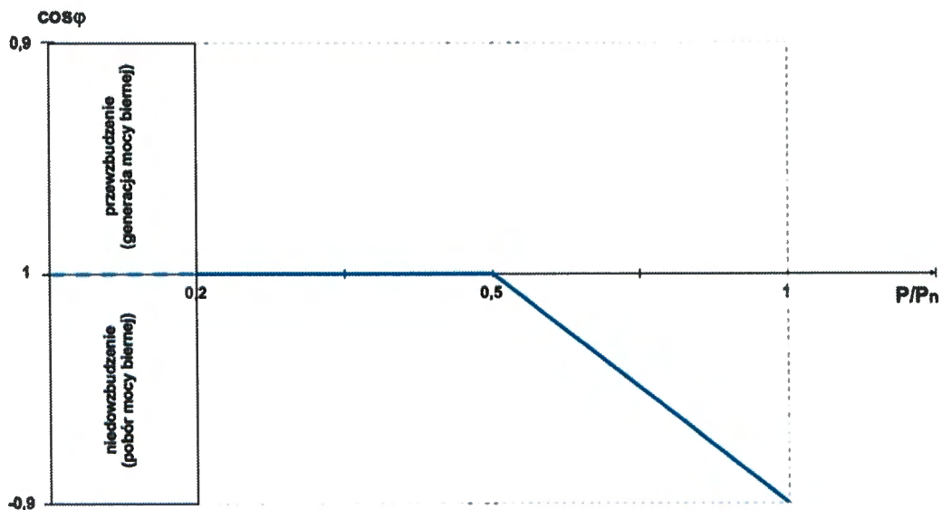
Rys. 5. Charakterystyka sterowania współczynnikiem mocy \cos \varphi w funkcji generowanej mocy czynnej wymagana przez ZEW Niedzica
