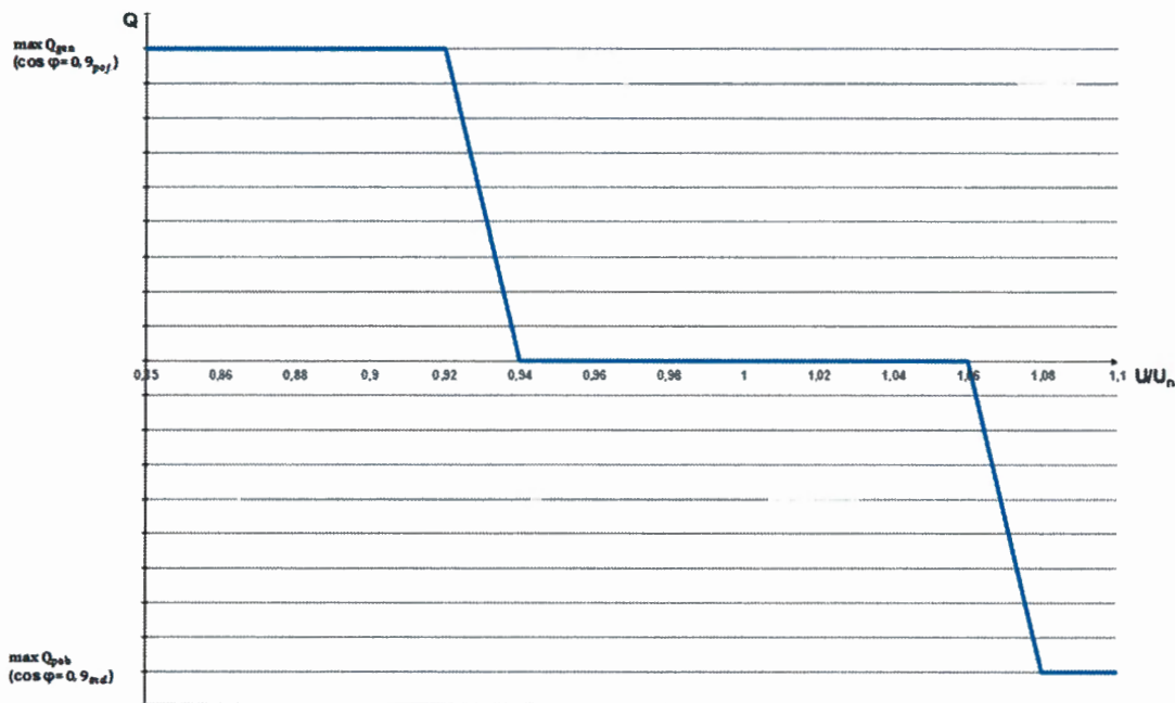
Rys. 3. Charakterystyka sterowania mocą bierną w funkcji napięcia wymagana przez ZEW Niedzica
